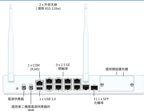
後視圖
