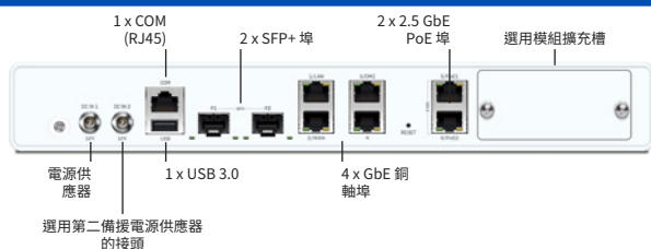
後視圖
