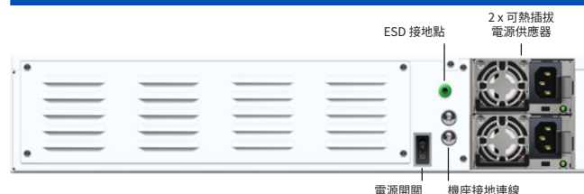
後視圖
