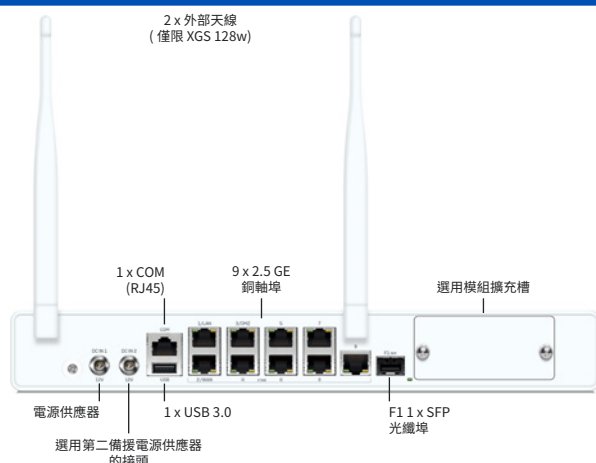
後視圖
